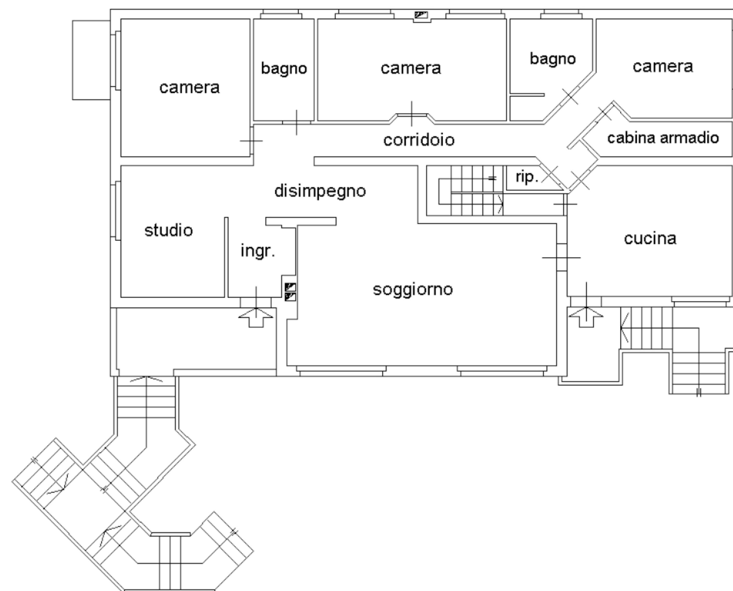
PRIMO PIANO H. 3.00
